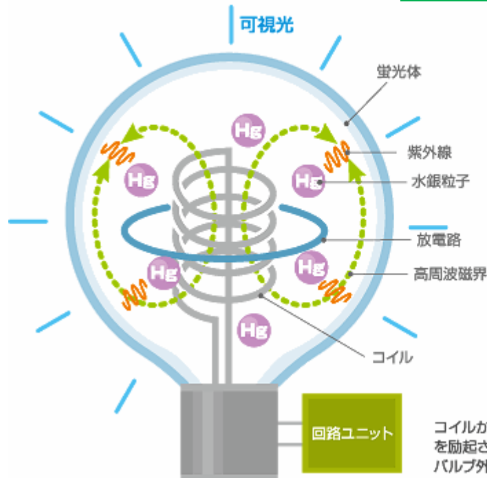
無電極ランプの構造(内巻コイル型)
