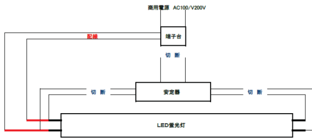
LED蛍光灯・器具内配線図(標準規格)
