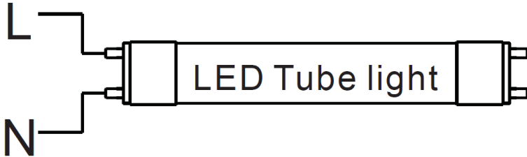
LED蛍光灯・器具内配線図(標準規格)
